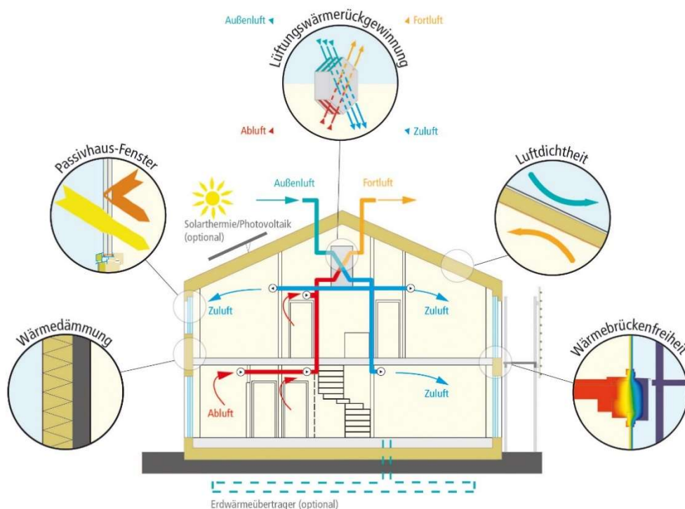
Abbildung 2: Die 5 Grundprinzipien eines Passivhauses (Quelle: IG Passivhaus)
